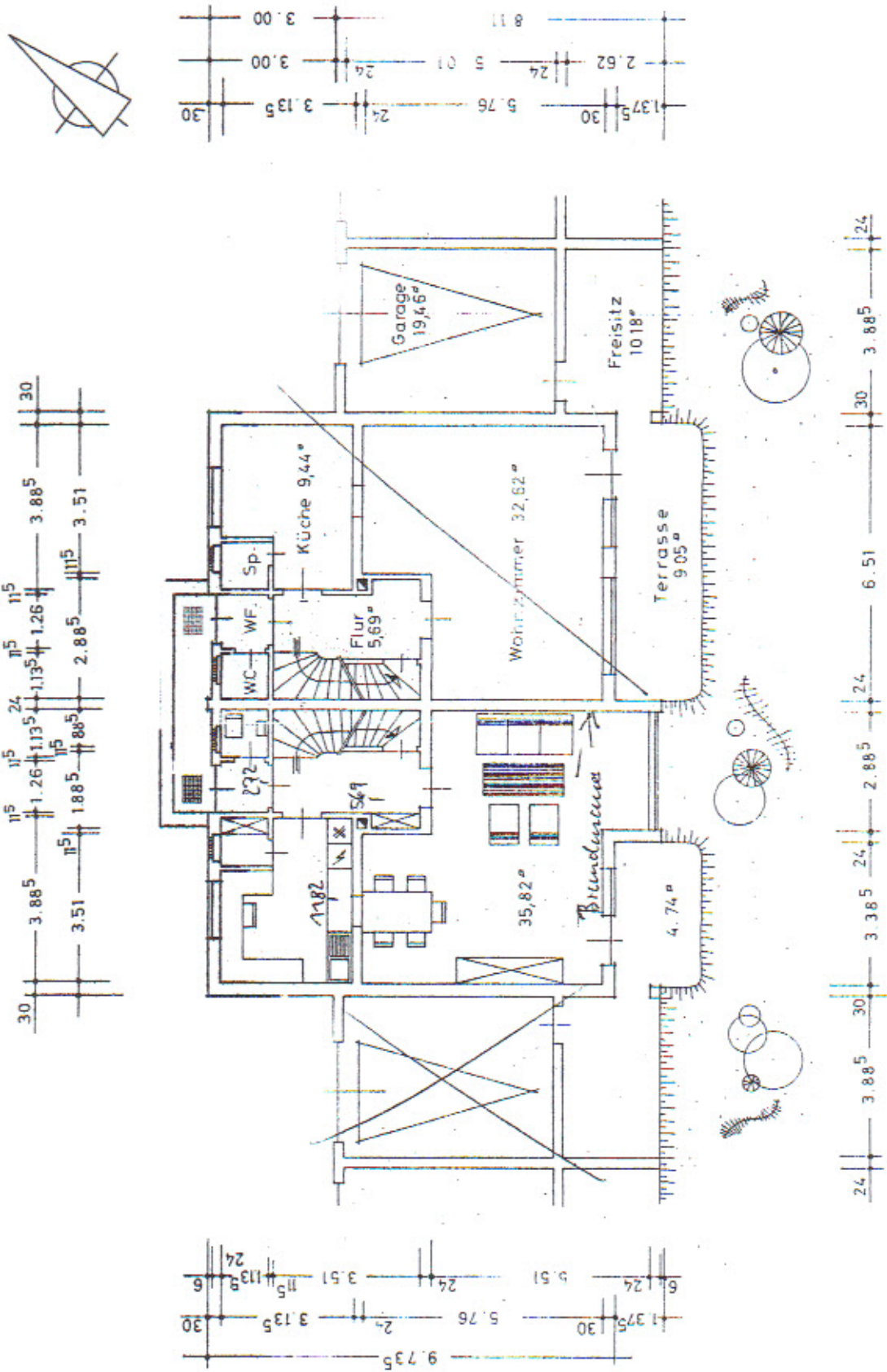
Grundriss Erdgeschoss DHH Hufschmiedstr. 10, Altötting 1
